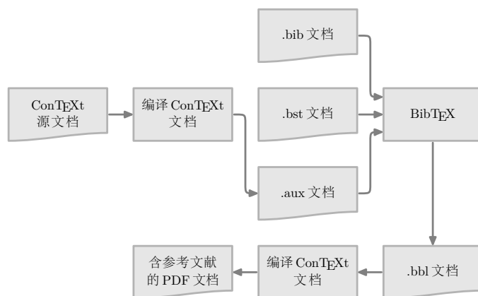
图 2 BibTeX 工作过程
